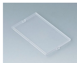
V6803200 Лицевая панель ПК (UL 94 V-0) прозрачный 67x42mm
