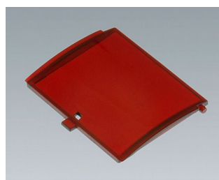
V6802302 Округлая передняя крышка на петлях ПК (UL 94 V-0) прозр. красная
