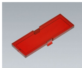
V6800300 Лицевая панель ПК (UL 94 V-0) прозр. красная 14x42mm
